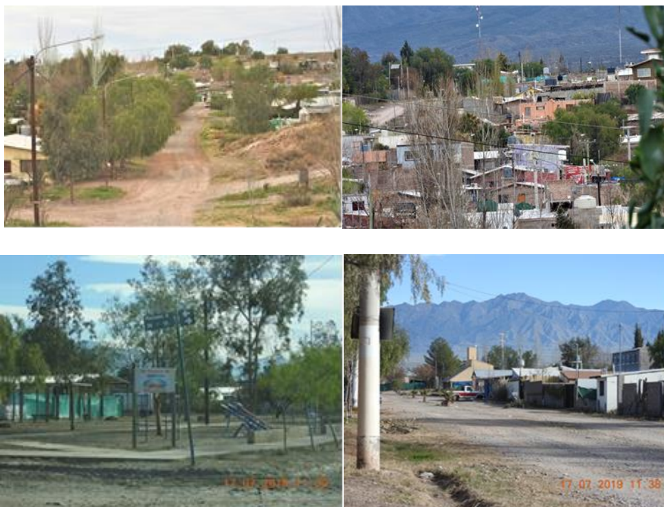
Figura N° 6: Piedemonte consolidado
