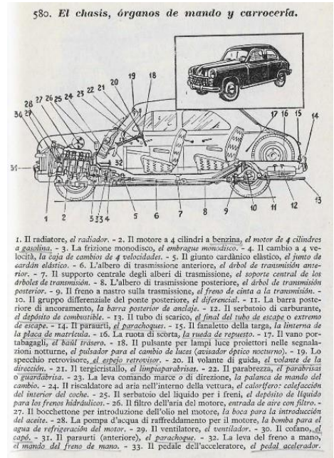
580. El chasis, órganos de mando y carrocería.
